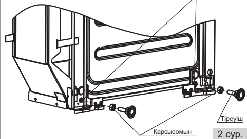
Реттелетін тіреуіштер орнатуға арналған орындар (төменгі жағынан көрініс)
