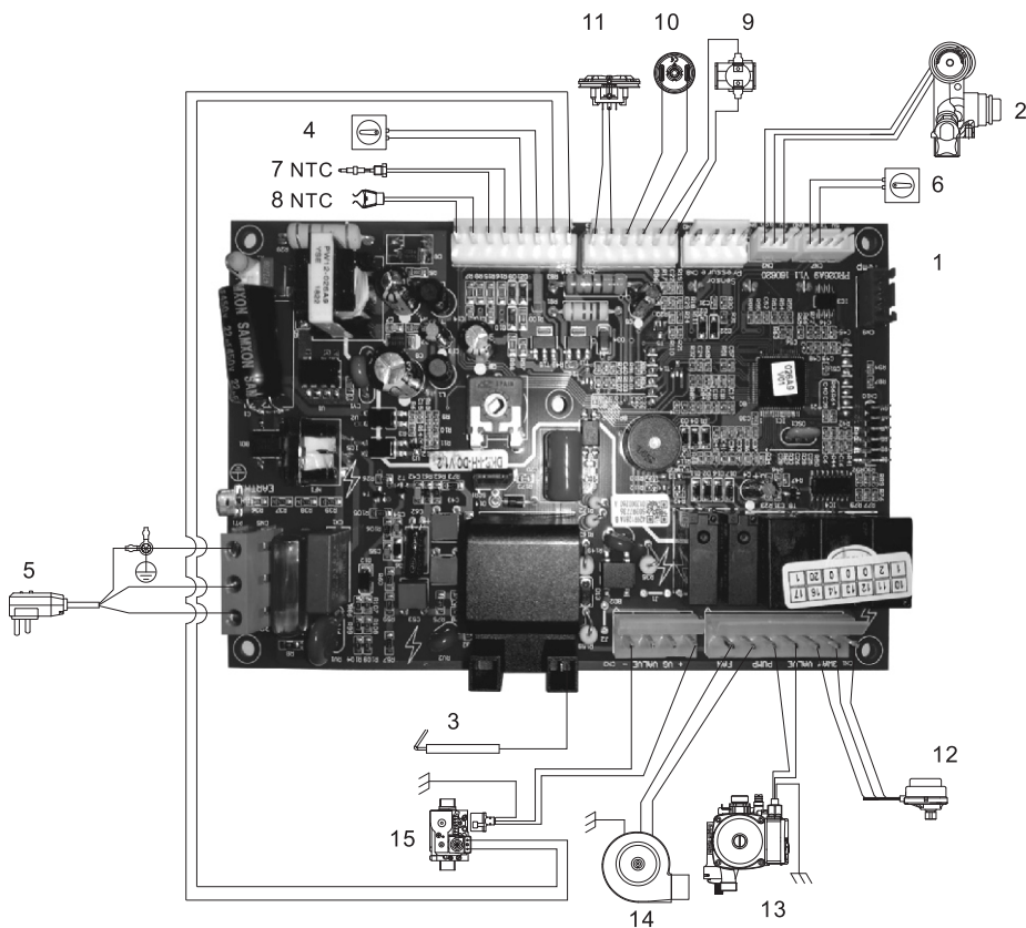
Схематическое изображение соединений газового котла
